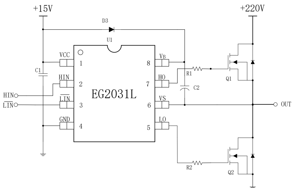
图 6-1. EG2031L 典型应用电路图
