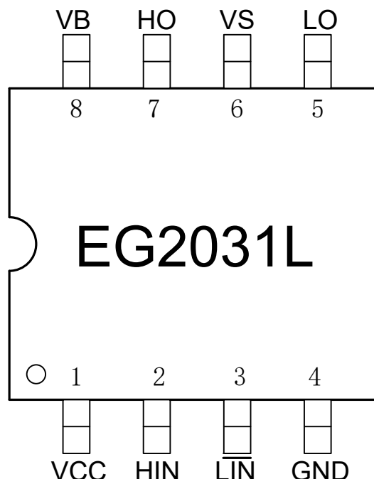
图 4-1. EG2031L 管脚定义
