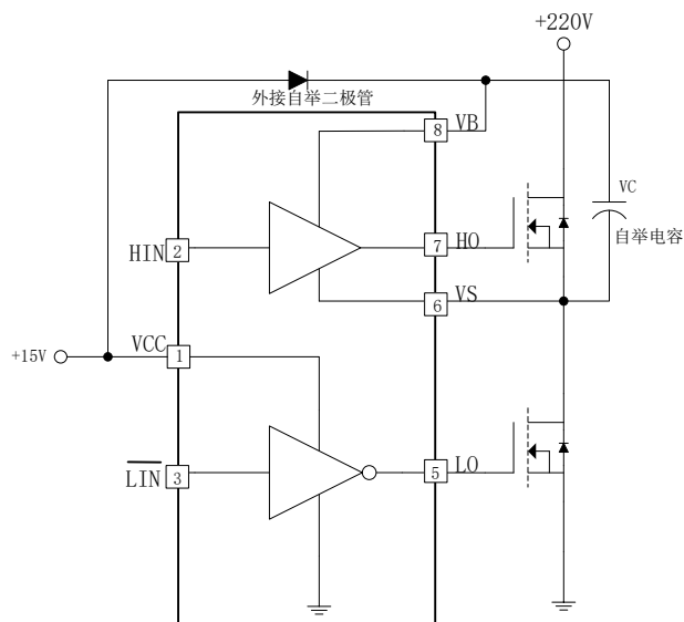
图 8-3. EG2031L 自举电路结构
