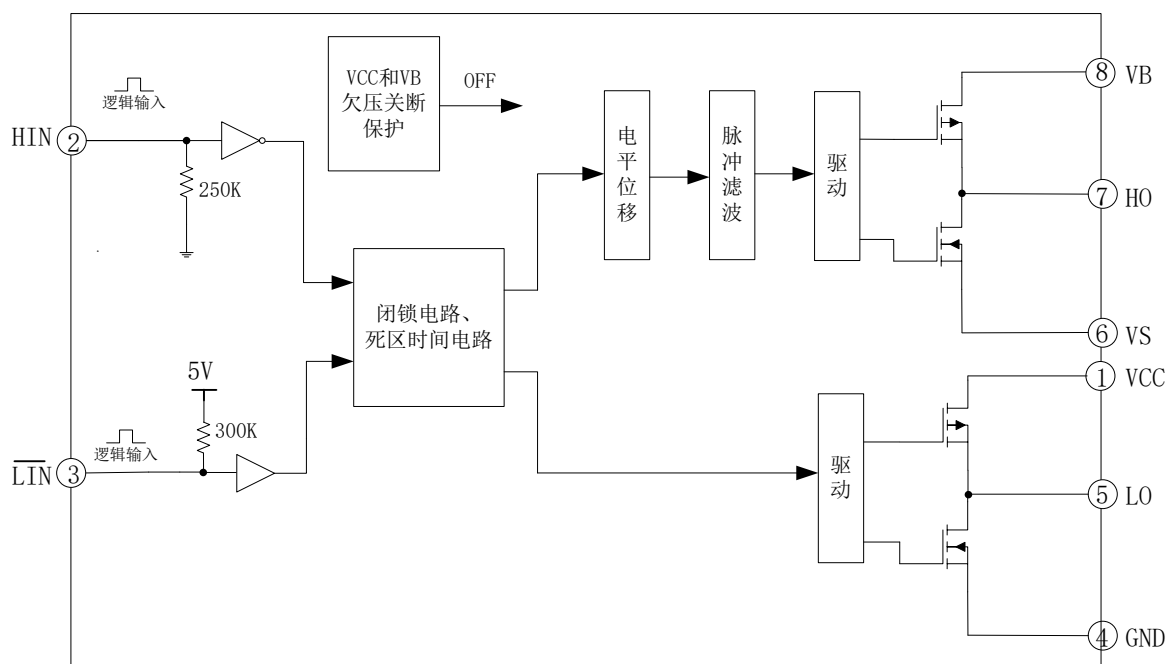
图 5-1. EG2031L 内部电路图
